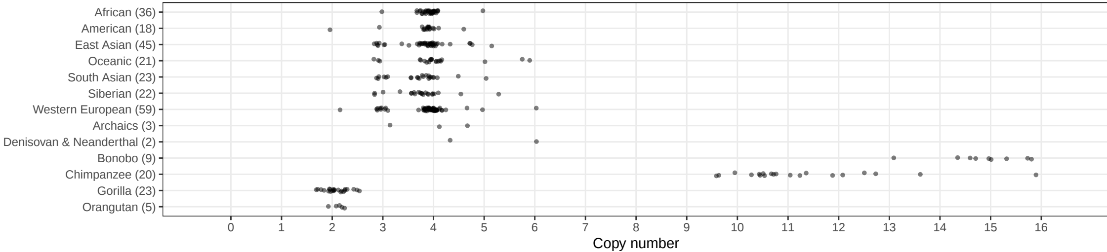
EIF3C_chr16:28688558-28735730_47172_hg38_hgdp_wssd
