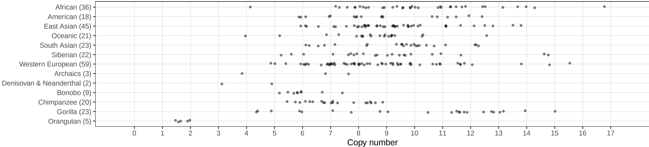
RASA4B_chr7:102482445-102517781_35336_hg38_hgdp_wssd
